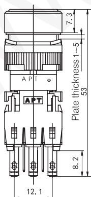
Round actuator
