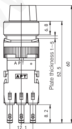
Round actuator
