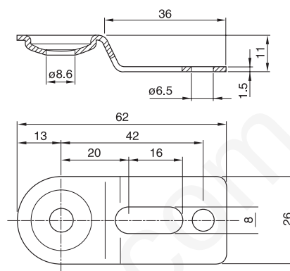
TG2 Hook
