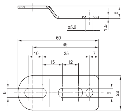
TG1 Hook
