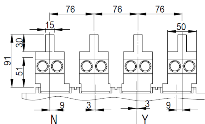
4 poles
