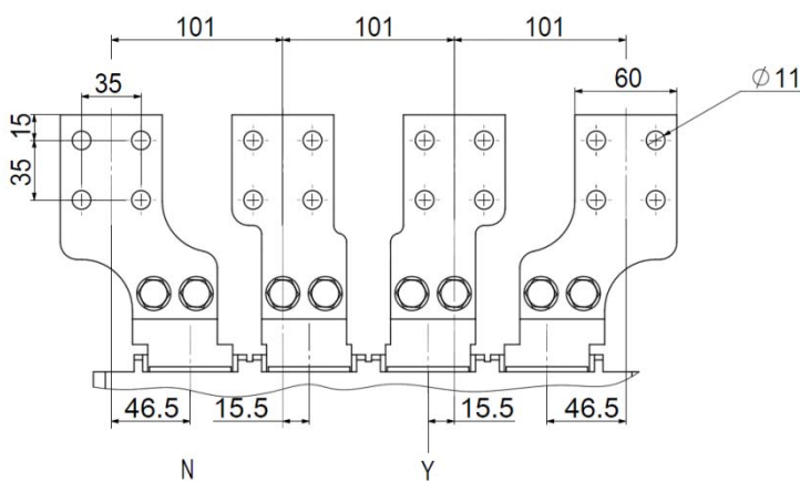
4 poles
